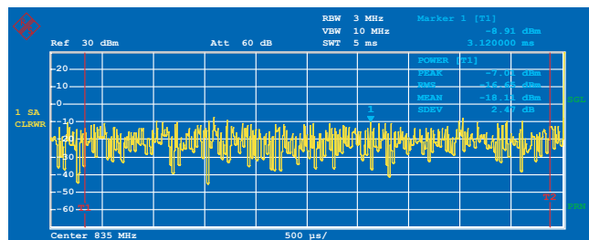
Messung der Burstleistung (oben)
