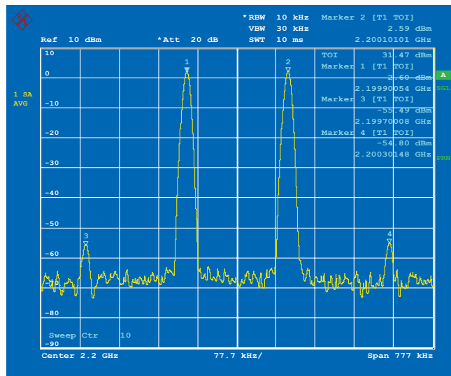
IP3-Messung
