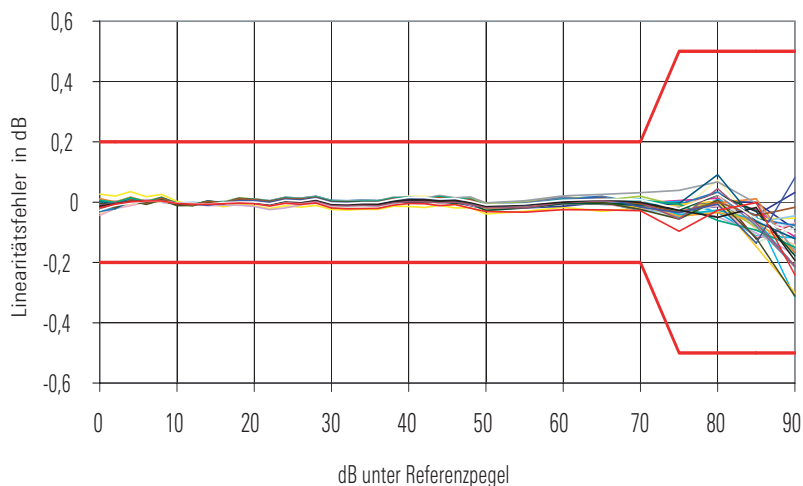
Anzeigelinearität bei ≤100 kHz Auflösebandbreite (Messung an 30 Geräten)
