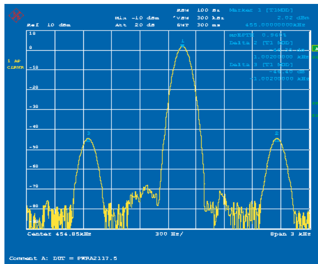
Messung des Modulationsgrads an einem AM-Signal
